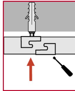
Deslizar la tapa en sentido longitudinal.
