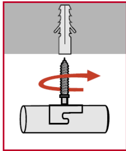
Atornillar con ayuda de un trozo de tubo.
